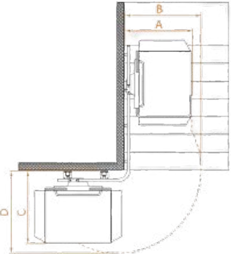
CALZADA CON CURVA DE 90º
