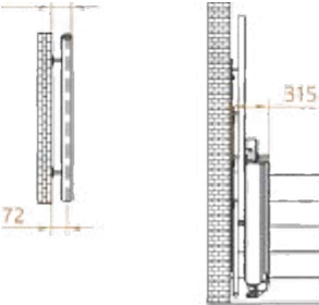
CALZADA MONTAJE EN PARED
