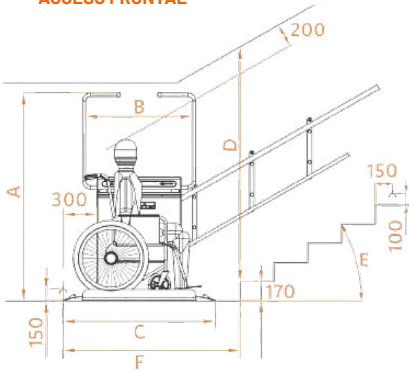
RAMPA DE ACCESO FRONTAL
